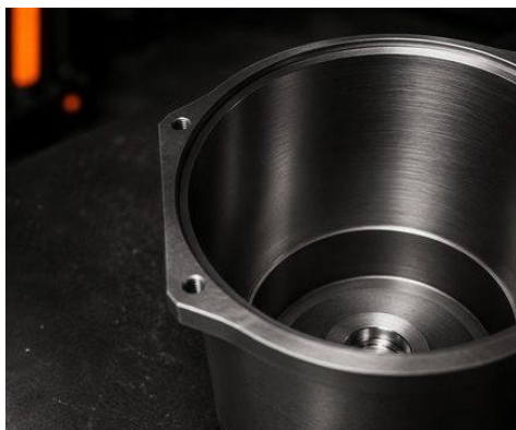
Präzisionsbearbeitung Graugussgehäuse
