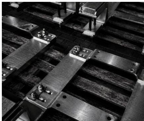
Gleisbefestigungselemente
