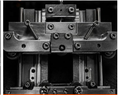
Fräsvorrichtung für Nutenfräsen
